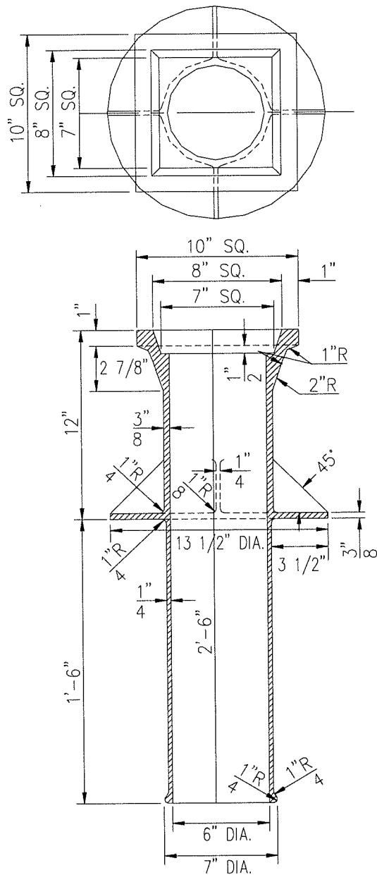
TOP NO. 3 & 4 (SQUARE COVER) EST. WT. 73 POUNDS
